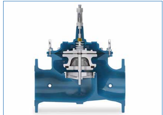
Vanne de base XG en coupe
