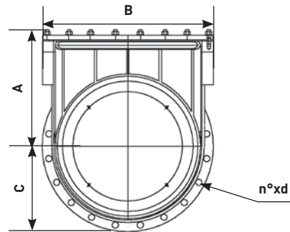
Version RSK DN 400 à 800
