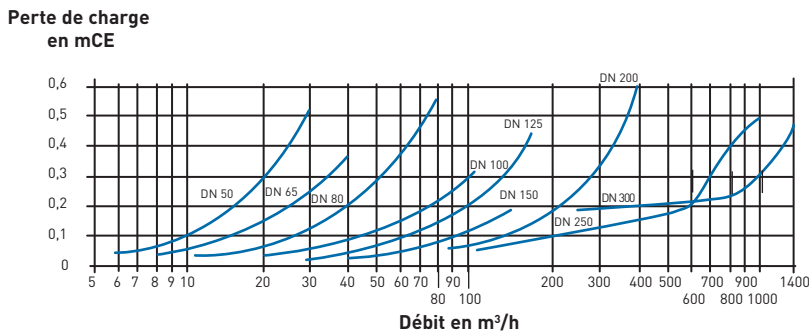
Courbes établies pour une eau à +20°C, clapet standard monté sur conduite horizontale.
