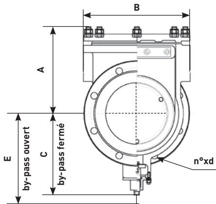
Version RSK-U DN 150 à 350
