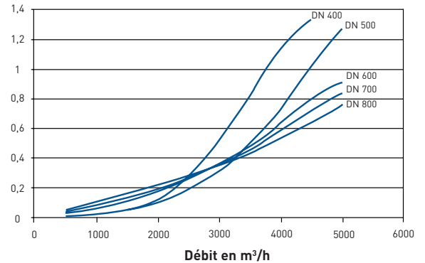
Courbes établies pour une eau à +20°C, clapet standard monté sur conduite horizontale.
