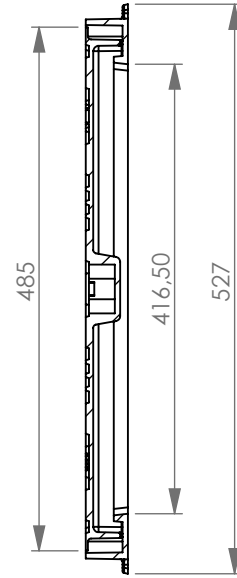
B-B (1 : 7)
